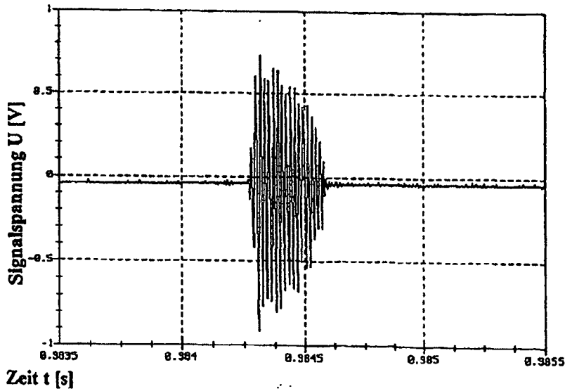
Schallemission spontaner kontinuierlicher Gelenkreibung
